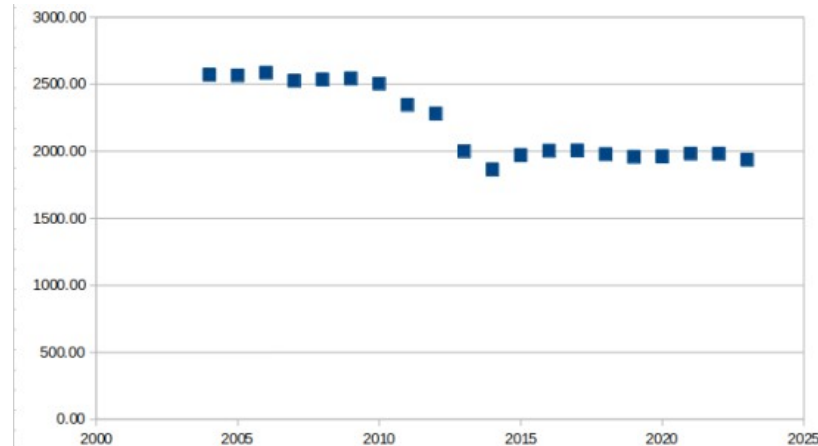
Fig. 1. Evolução do salário líquido para um professor, exemplo com o índice 195.
